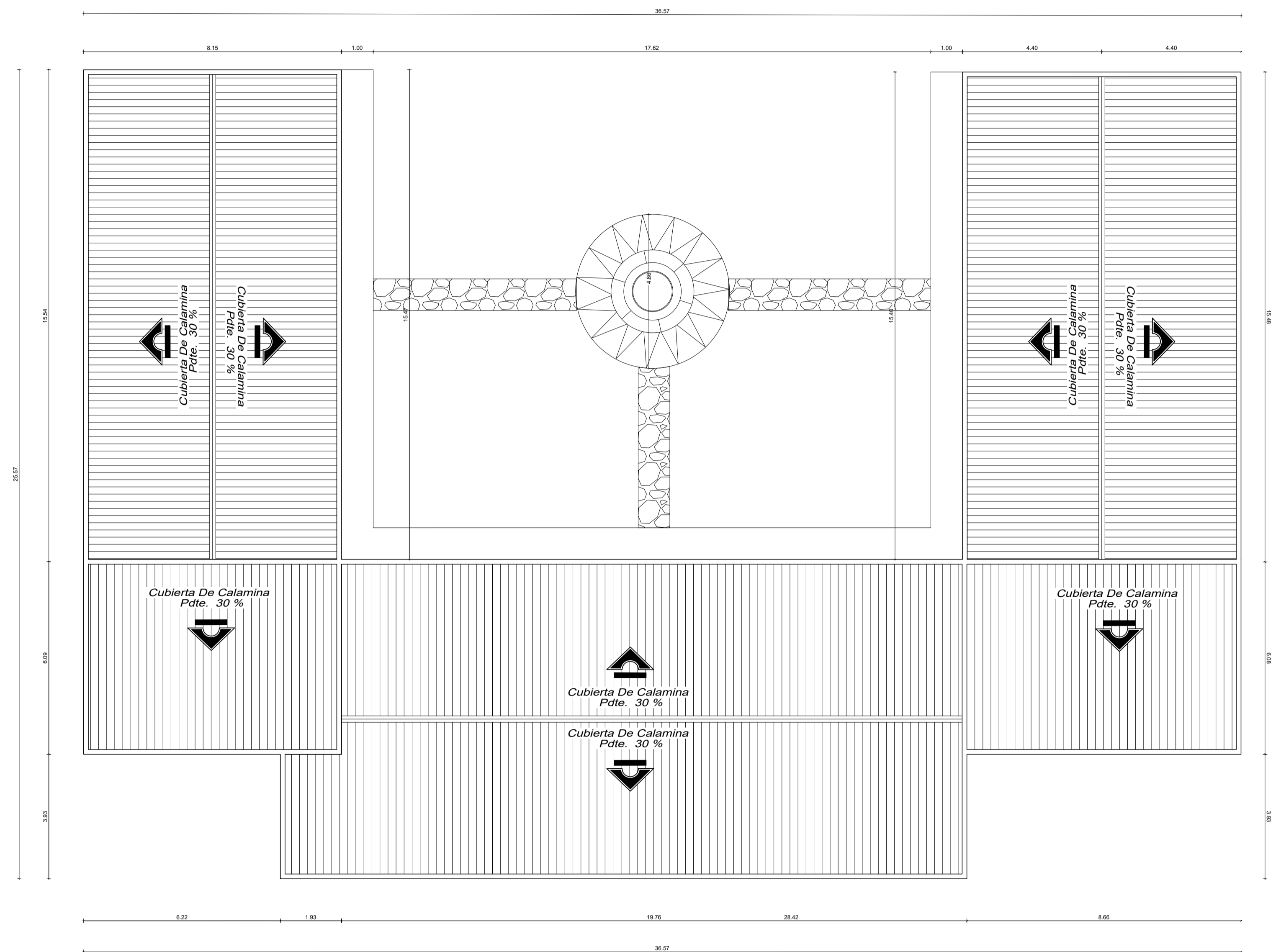
PLANO DE TECHOS
